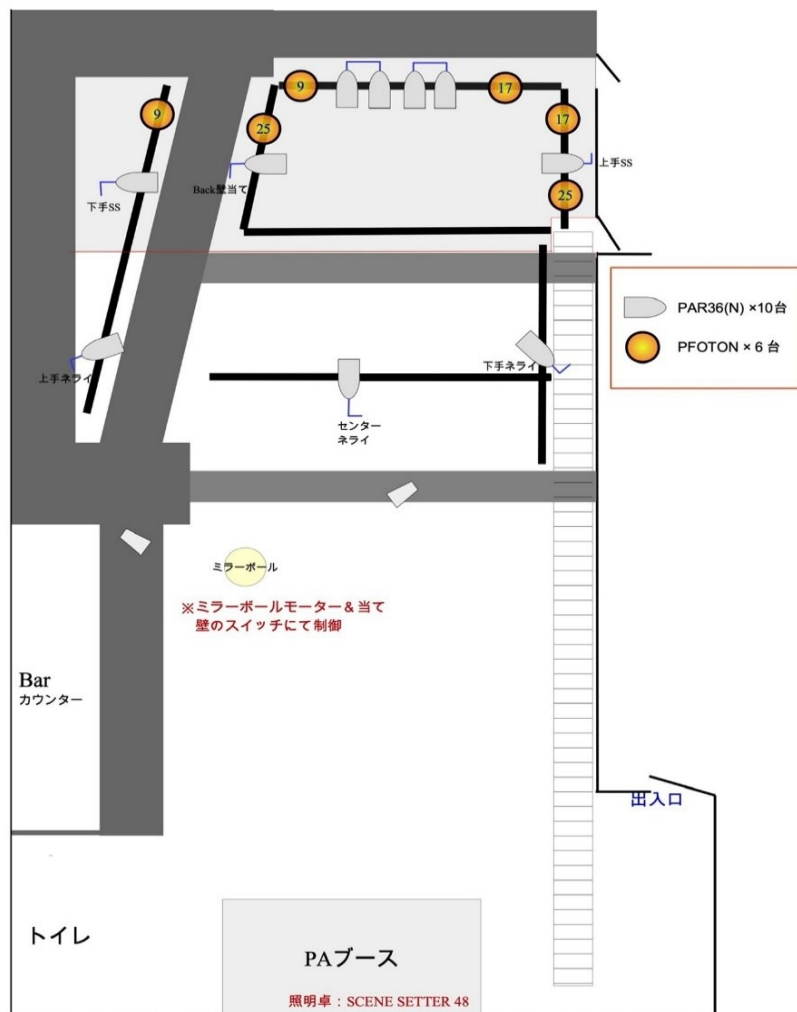
照明仕込図 図3
