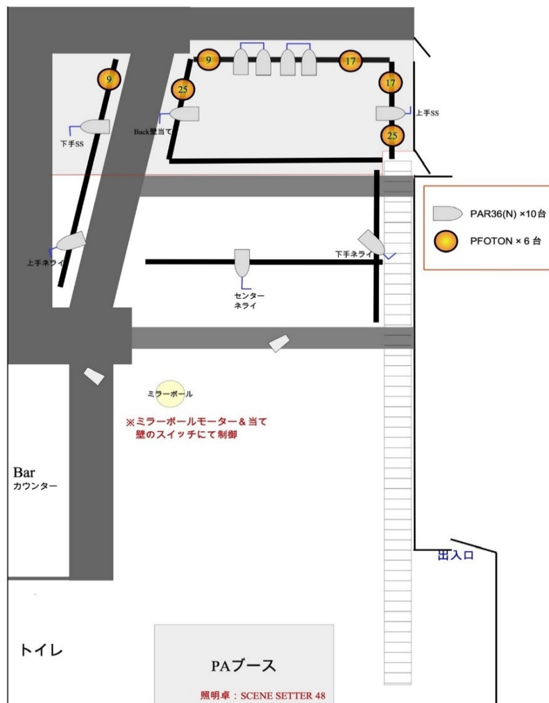
照明仕込図 図3
